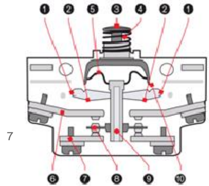
Рис. 1 Механизм работы выключателя
